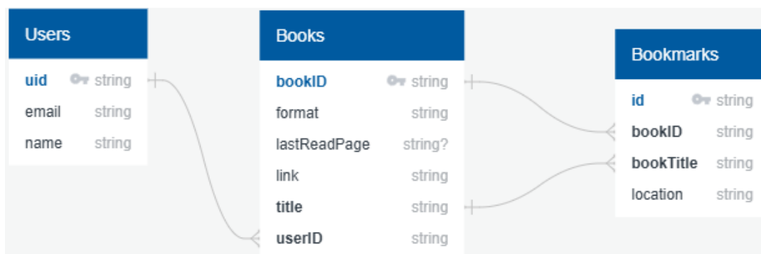
Hình 4.1: Sơ đồ Cơ sở dữ liệu của ứng dụng
