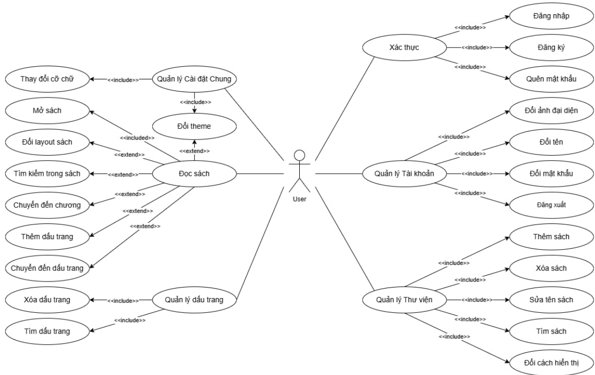
Hình 2.1: Sơ đồ Use-case
