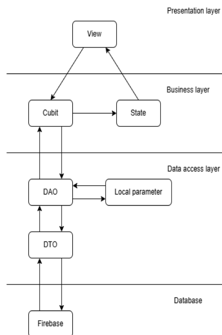
Hình 3.2: Phân lớp kiến trúc Dart
